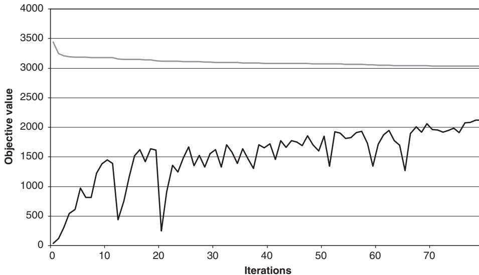
Fig. 4. Standard ColGen(t) : LB = 2121.40.
